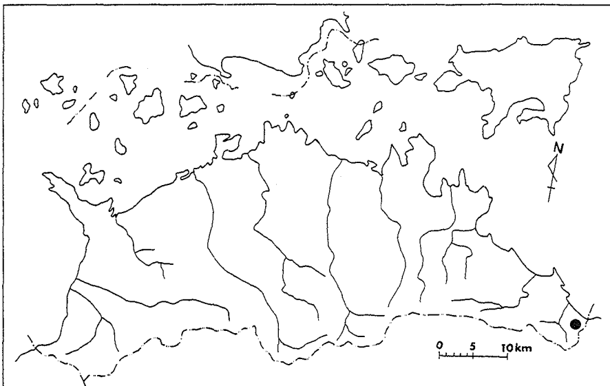
図 1. 香川県における Fredericella sultana の産地。
