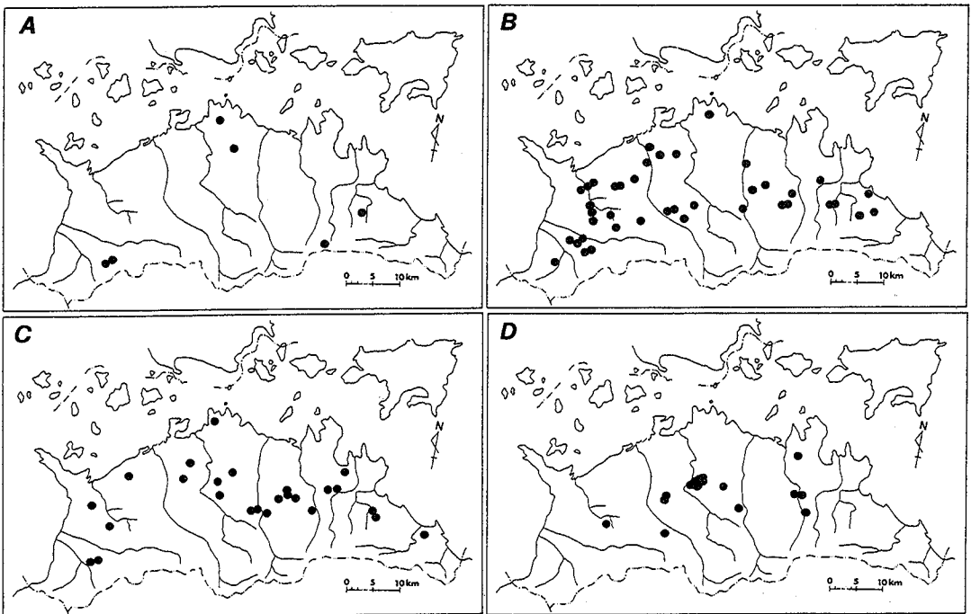
図2. 淡水苔虫4種の分布図(久米, 1999 に加筆した).
